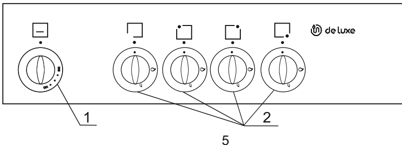
Панель управления плит модели 5040.54г-000
